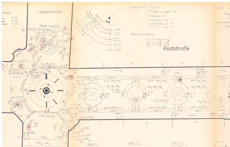
Lageplanauszug Neugestaltung Poststraße 1988
