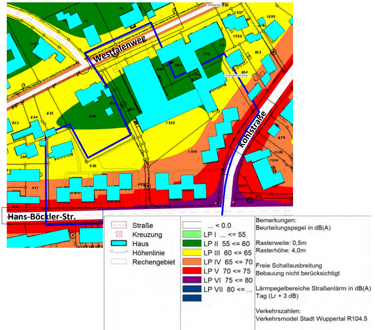
Abbildung 8: Straßenverkehrslärm, Berechnung nach DIN 4109, tags
