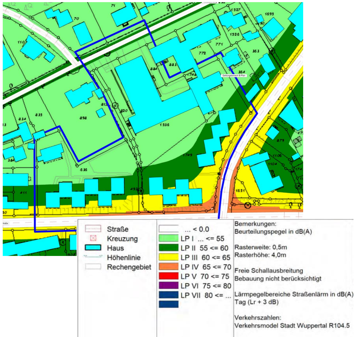
Abbildung 9: Straßenverkehrslärm, Berechnung nach DIN 4109, nachts
