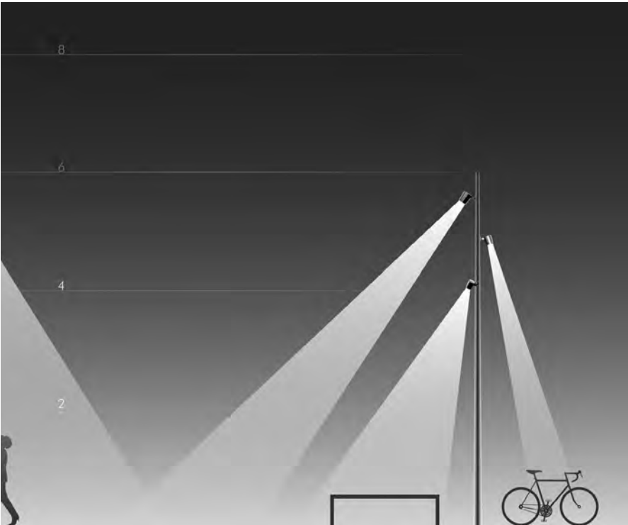
Produktbeispiel eines „Multistrahlersystems“. Mehrere Leuchtenköpfe können je nach Nutzung individuell ausgerichtet werden und unterschiedliche Optiken aufweisen.
