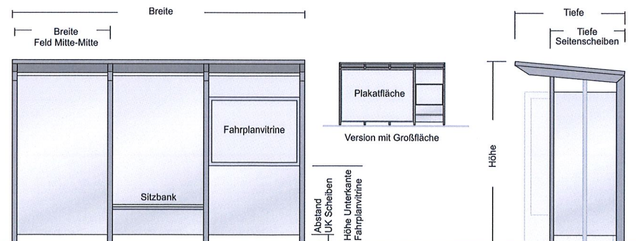
Technische Zeichnung M 1:50
