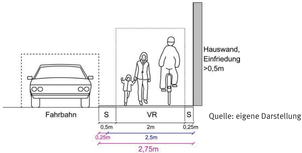
Abb. 29: Erforderliche lichte Breite eines gemeinsamen Geh- und Radwegs (innerorts) entlang einer Fahrbahn mit Längsparkständen
