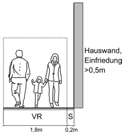
Abb. 9: Mindestbreite für Fußweg in Wohngebieten geringer Dichte (bis 3 Geschosse)*
