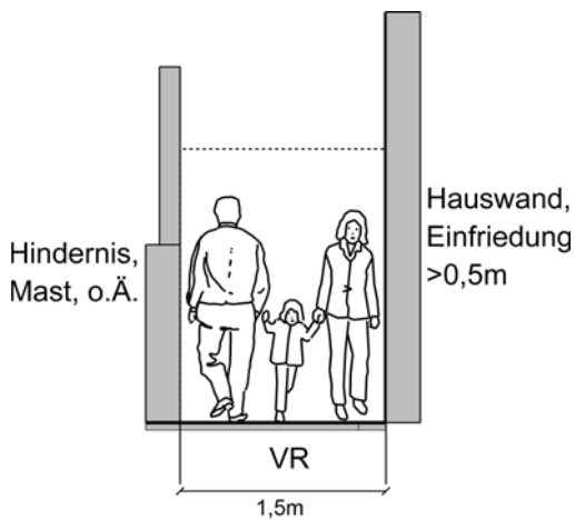
Abb. 11: minimale Engstelle für Fußgängerkehr (max. 50m Länge)
