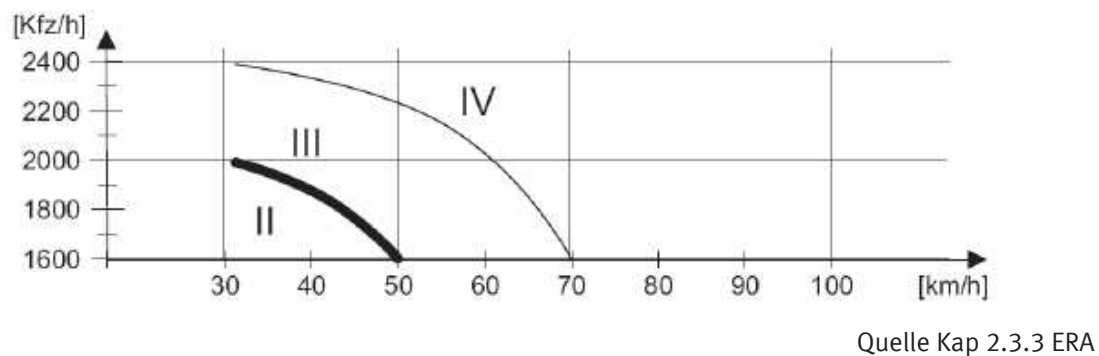
Abb. 4: Bemessungstabelle vierstreifige Straßen mit zwei getrennten Richtungsfahrbahnen (Fahrbahnbreite \geq 7\text{m} )
