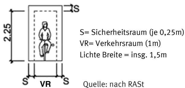
Abb. 14: Verkehrsraum und Sicherheitsraum eines Radfahrers
