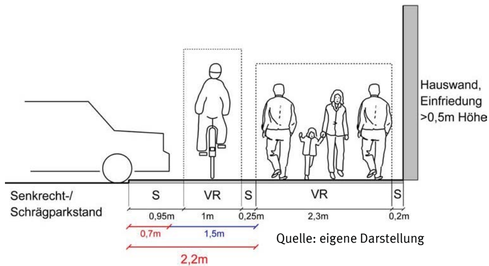
Abb. 19: Erforderliche lichte Breite eines Einrichtungsradwegs (ohne Überholmöglichkeit) entlang einer Fahrbahn mit Senkrecht- und Schrägparkständen (bis 50 gon)
