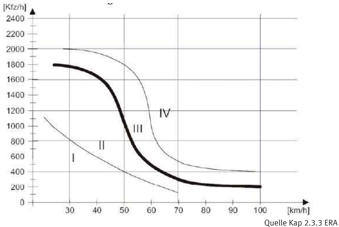
Abb. 3: Bemessungstabelle zweistreifige Straßen (Fahrbahnbreite \geq 7\text{m} )
