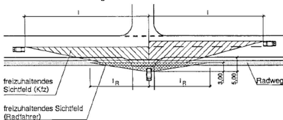
Abb.35: Anfahrtssicht auf Radweg aus einmündendem Kraftverkehr
