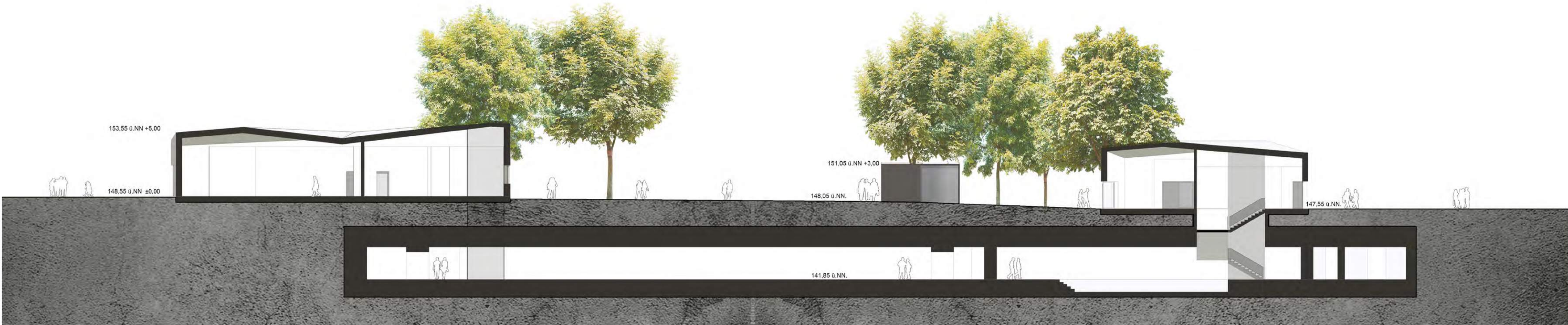
Geländeschnitt 1_200
