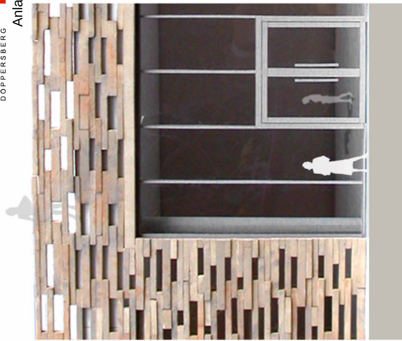
TEILANSICHT NATURSTEIN-/GLASFASADE M 1:20
