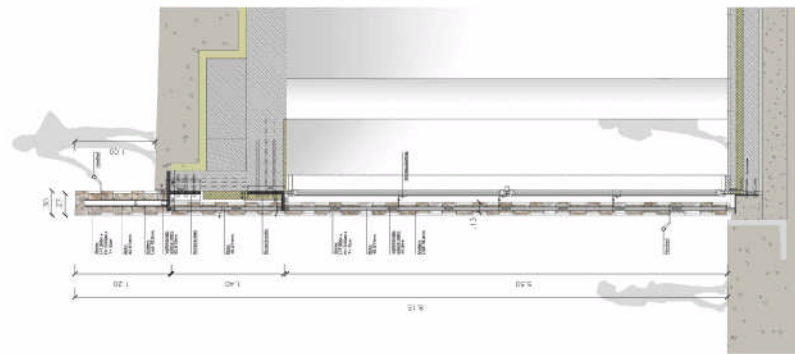
SCHNITT LADEN NATURSTEINFASADE M 1:20
