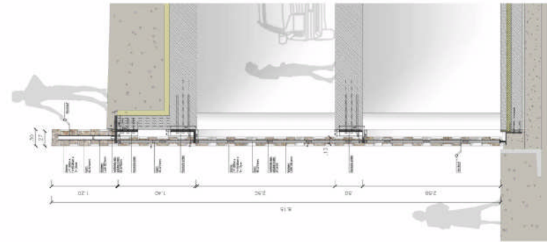
SCHNITT PARKDECK M 1:20
