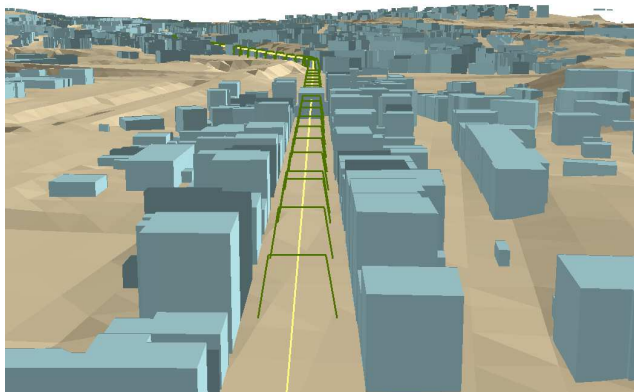
Digitales Lärmmodell und Ergebnis der Berechnungen
