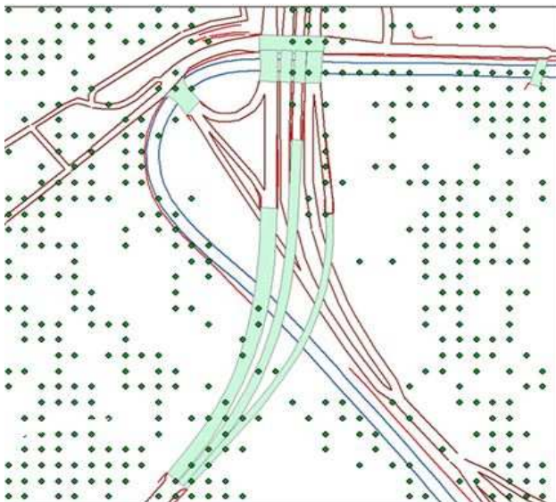
Ausgedünntes Geländemodell und künstliches Geländemodell einschließlich Straßen, Lärmschutz, Mauern und Bebauung
