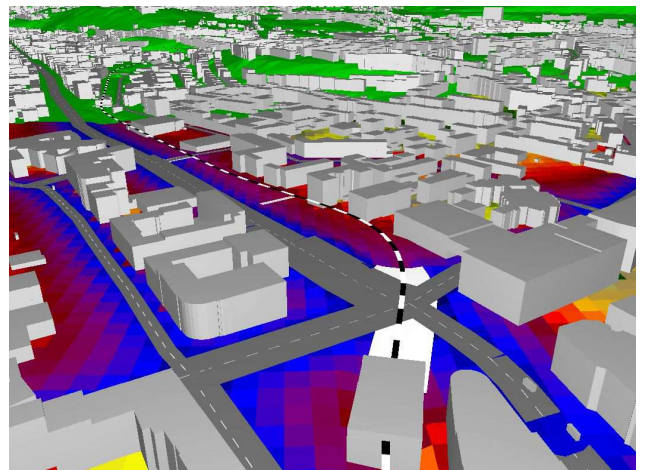
Digitales Lärmmodell und Ergebnis der Berechnungen
