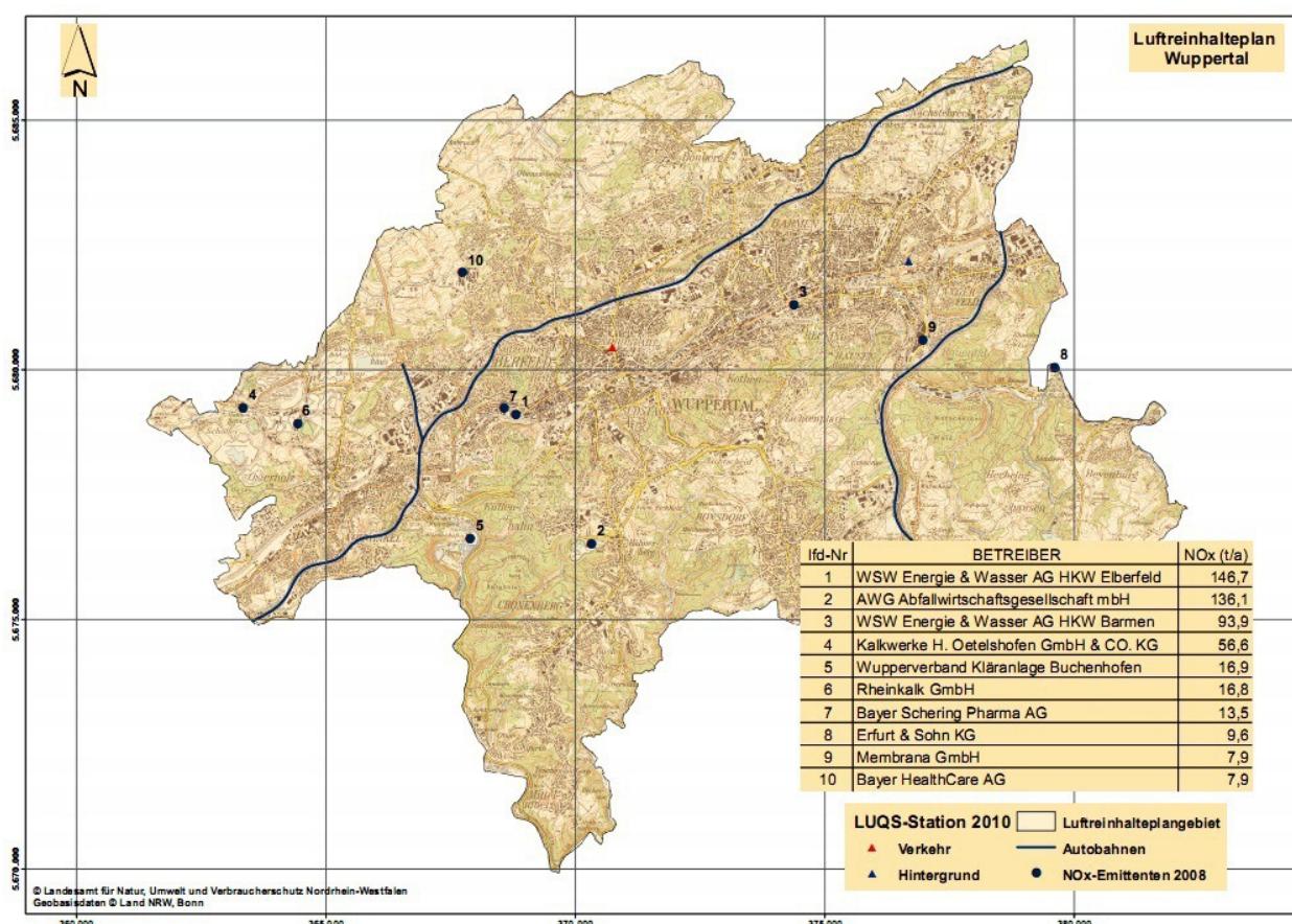
Abb. 3.2.3/3: Stickstoffdioxid ( \text{NO}_x )-Emissionen der nach dem BImSchG genehmigungspflichtigen Anlagen der Industrie im Luftreinhalteplan Wuppertal
