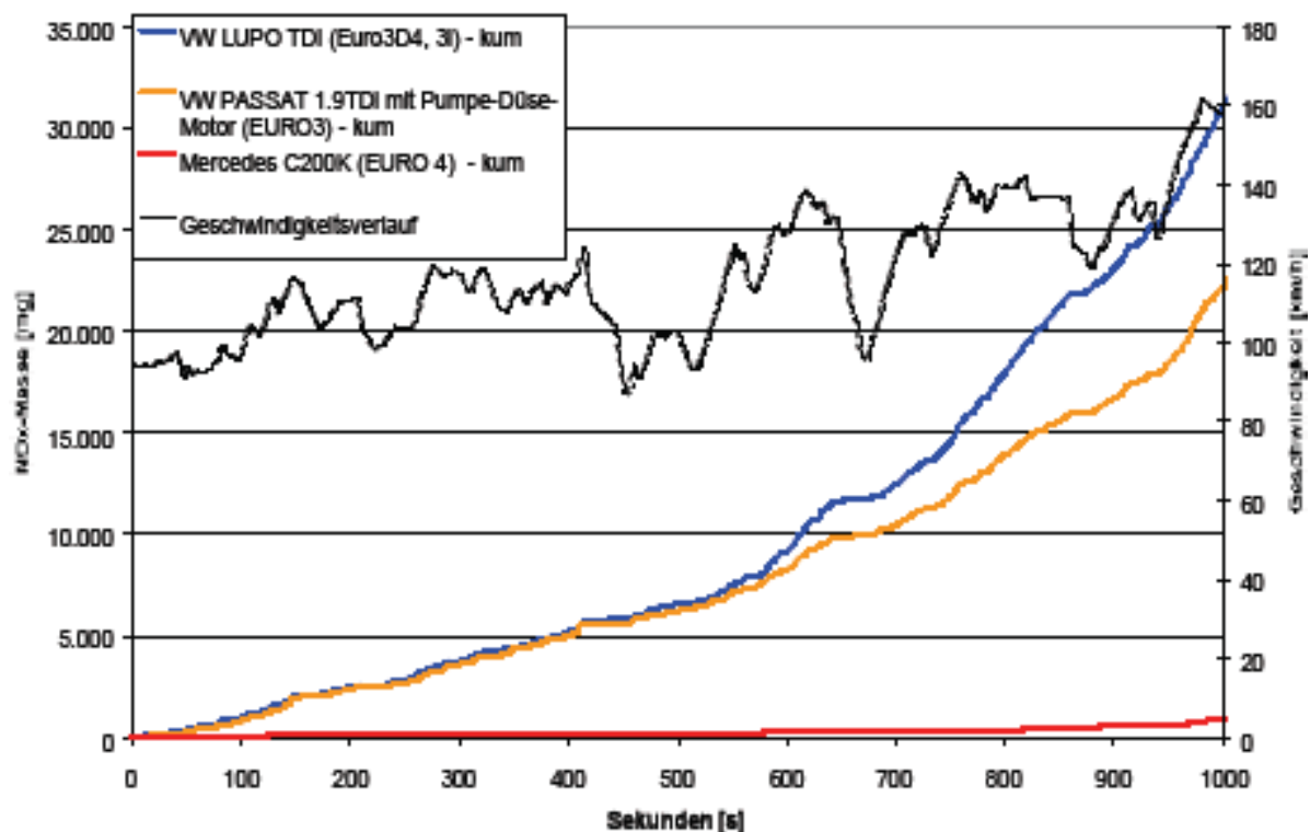
Abb. 7.1/1: Kumulierte NO x -Emissionen von zwei Diesel Pkw im Vergleich mit einem Otto Pkw in einem Autobahnzyklus, der bis 160 km/h reicht 43
