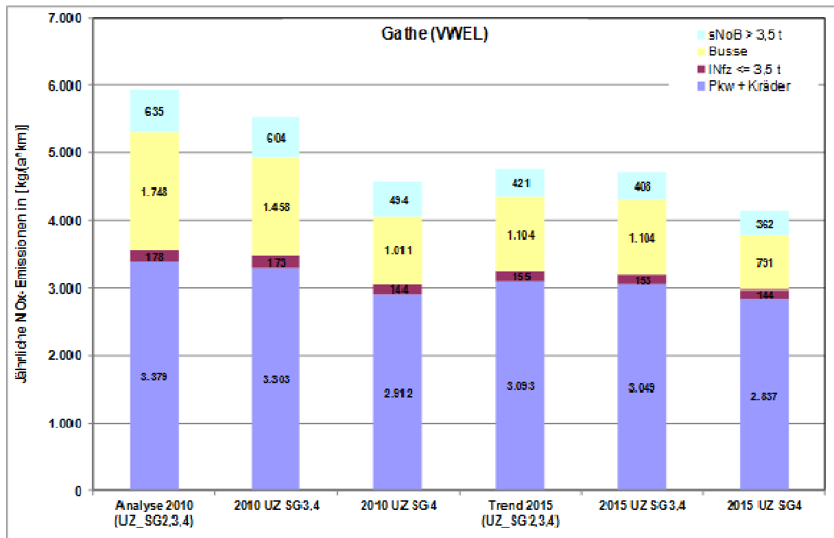
Abb. 6.1/1: \text{NO}_x -Emissionsanteile verschiedener Fahrzeugarten für Wuppertal Gathe, Analyse 2010, Trend 2015 und Maßnahmen (UZ=Umweltzone, SG=Schadstoffgruppe)
