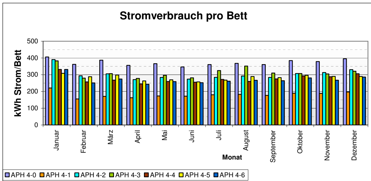
Abb. 2: Stromverbrauch in 7 Einrichtungen des Eigenbetriebs Altenpflege und Altenpflegeheime für das Jahr 2007
