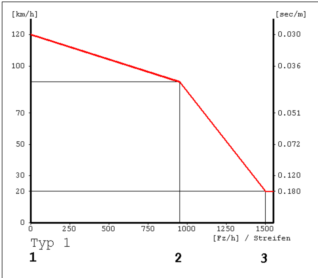
Abbildung 3: Widerstandsfunktionen in PSV (Quelle: Softwarekontor Helmert Hilke)
