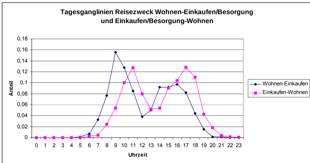
Abbildung 38: Tagesganglinien Einkaufsverkehre (nah) und Besorgungsverkehre
