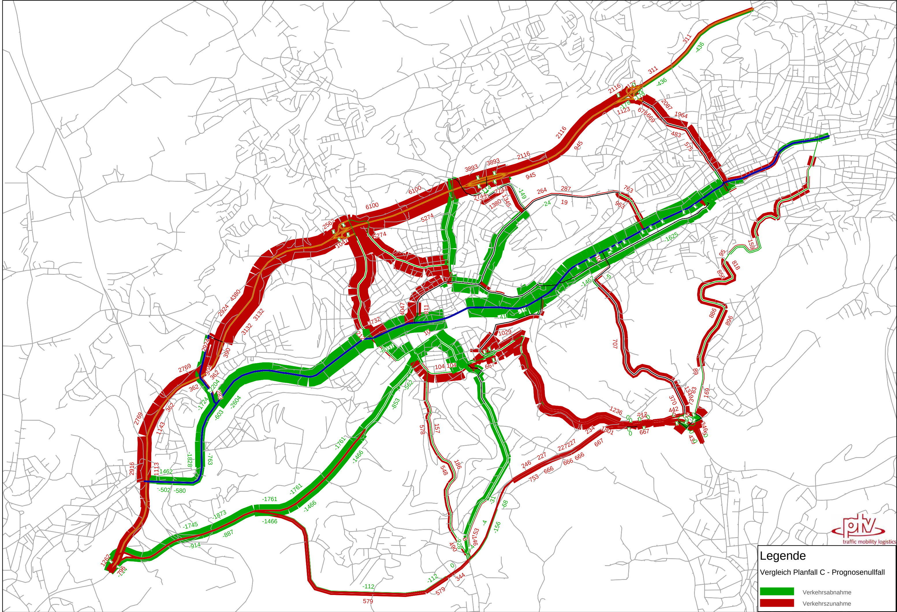
Planfall C - Differenzbelastungen zu Prognosenullfall (großräumig)
