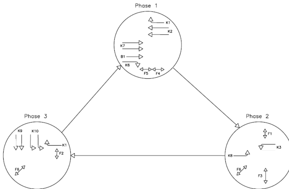
Abbildung 28: möglicher Phasenfolgeplan, LZA 223 Robert-Daum-Platz
