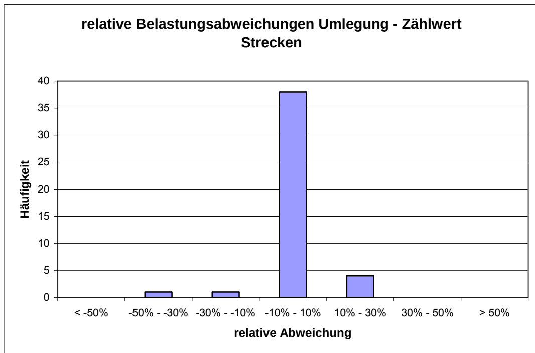
Abbildung 5: Relative Belastungsabweichung Strecken
