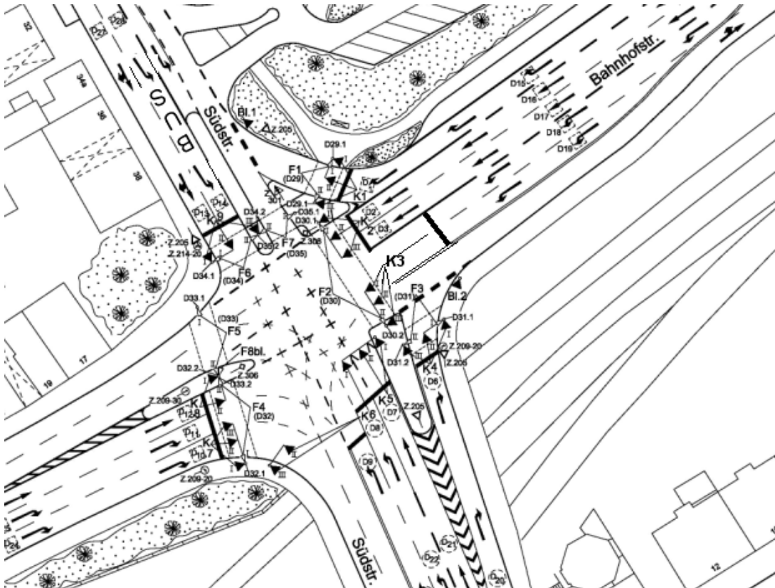
Abbildung 32: Signallageplan LZA 232, Südstraße/Hoeftstraße/Bahnhofstraße
