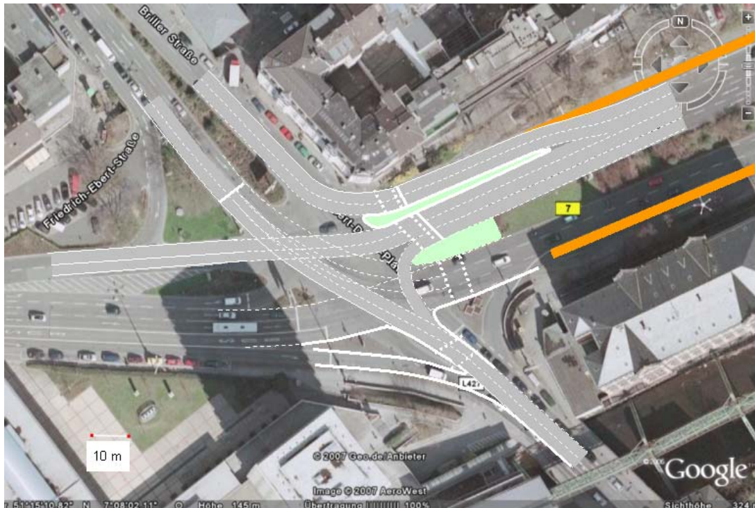
Abbildung 27: Schematische Gestaltungsskizze LZA 223 Robert-Daum-Platz
