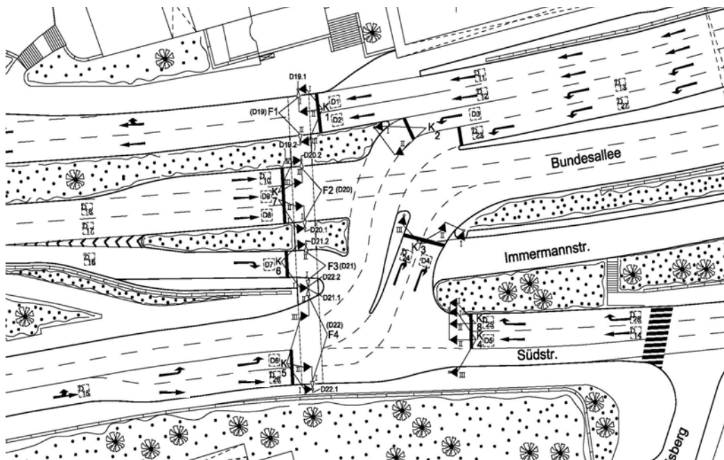
Abbildung 34: Signallageplan LZA 257, Bundesallee (B7)/Südstraße (bisherige Planung)
