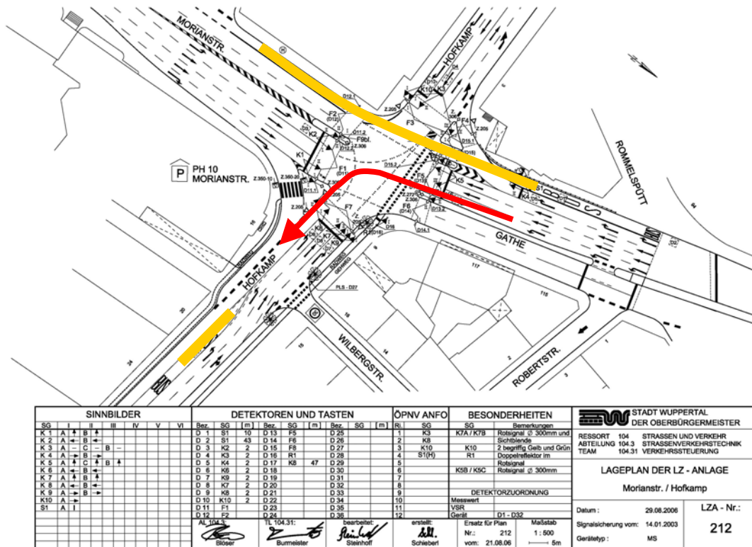
Abbildung 23: Signallageplan LZA 212, Morianstraße/Hofkamp
