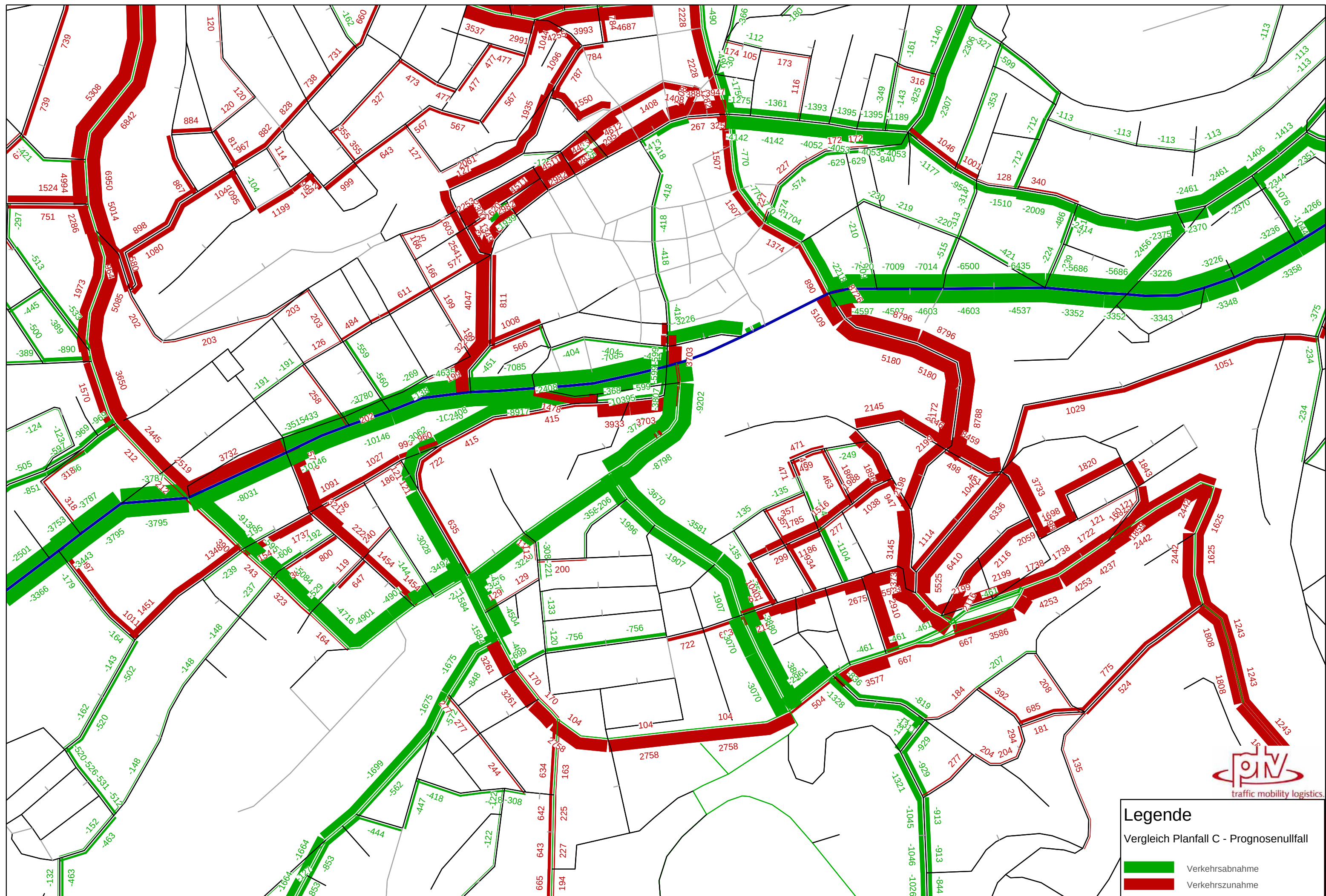
Planfall C - Differenzbelastungen zu Prognosenullfall
