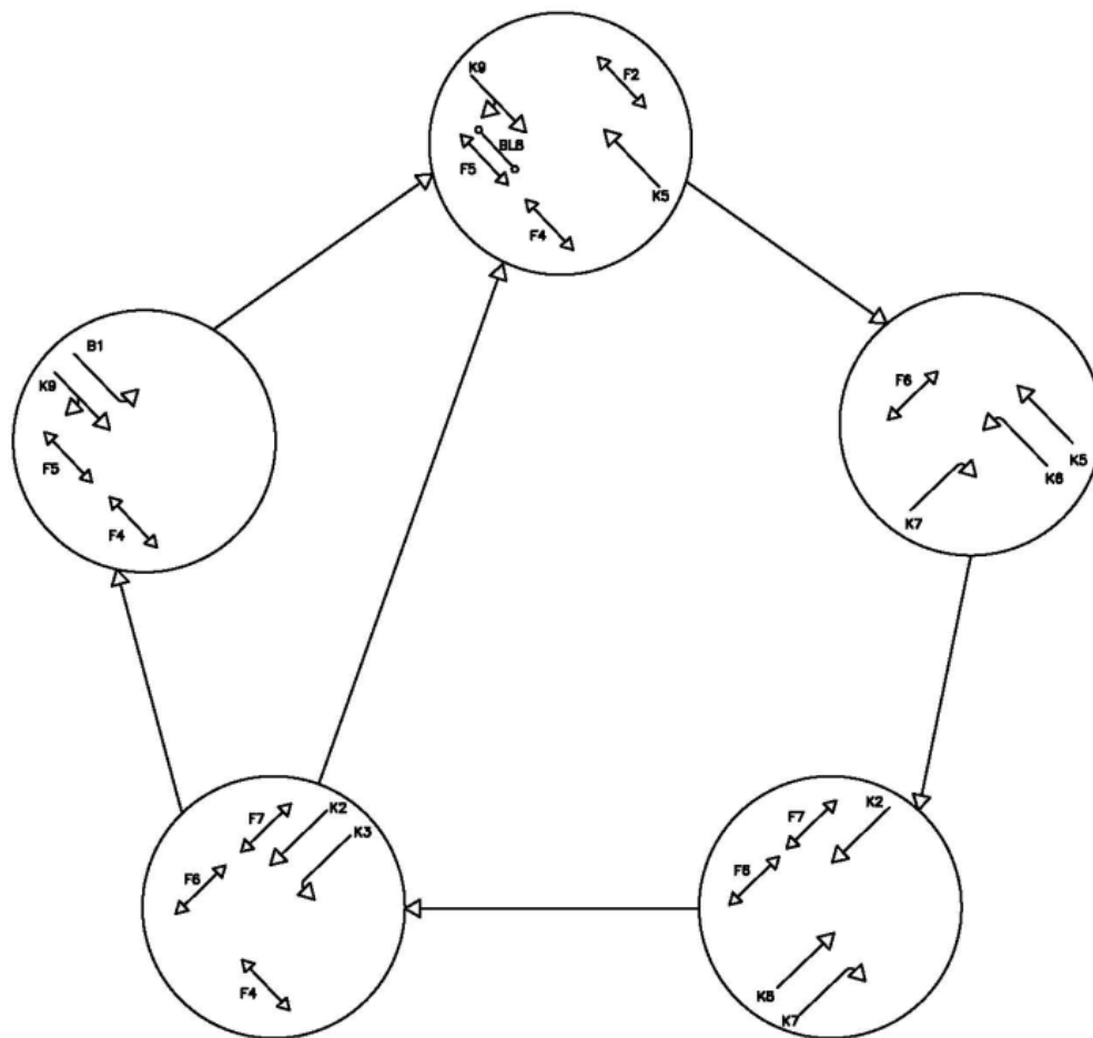
Abbildung 33: Phasenfolgeplan, LZA 232, Südstraße/Hoeftstraße/Bahnhofstraße
