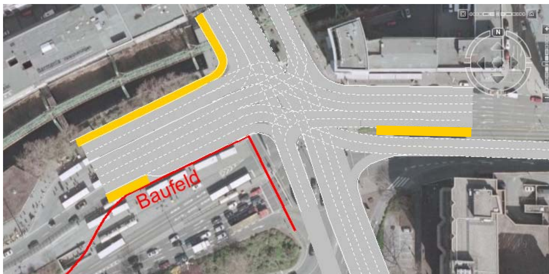
Abbildung 24: Schematische Gestaltungsskizze LZA 214, Brausenwerth
