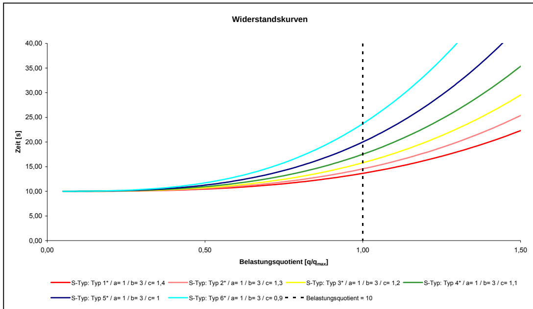
Abbildung 4: Widerstandsfunktionen in VISUM für unterschiedliche Streckentypen
