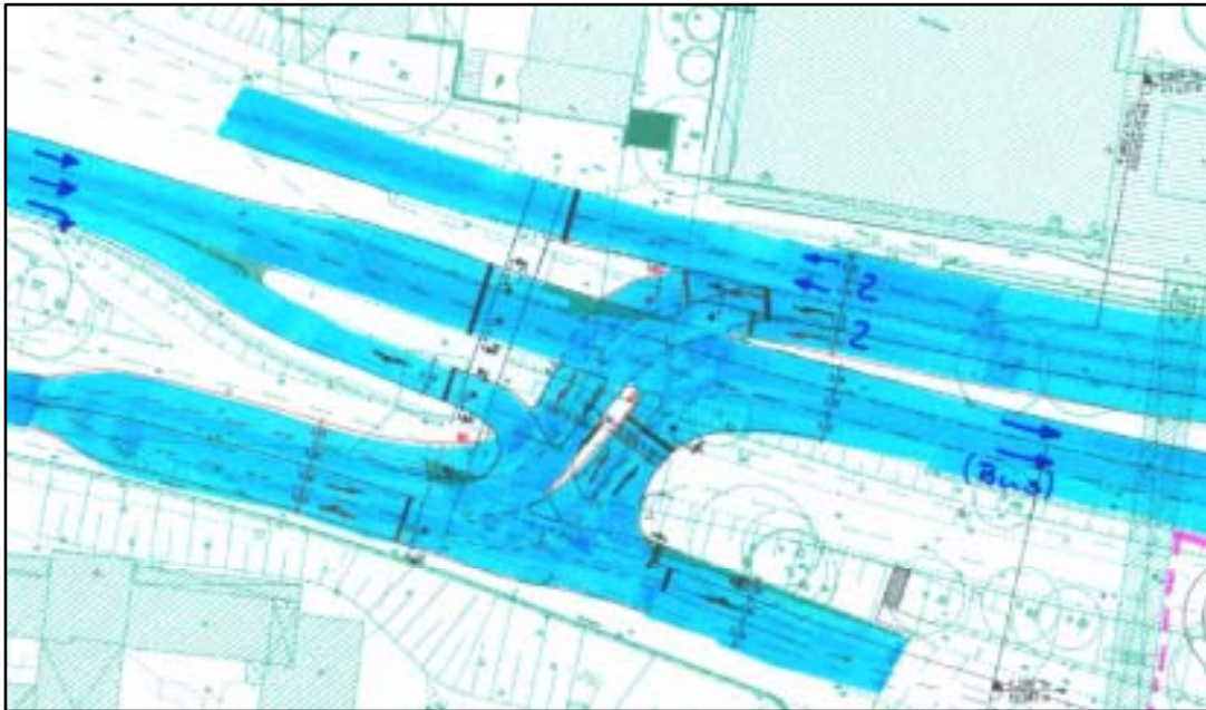
Abbildung 10: Plandarstellung Vollanschluss Südstraße - Bundesallee
