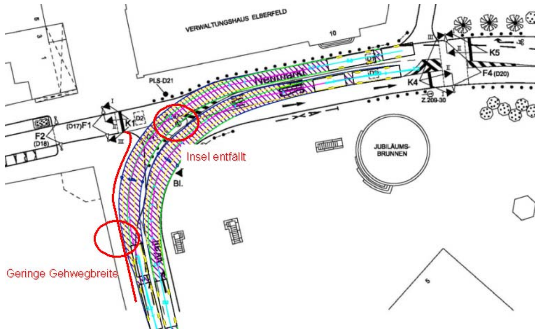
Abbildung 26: Signallageplan LZA 216 Neumarkt/Wall/Rommelspütt (Baustellenzustand Hertie)
