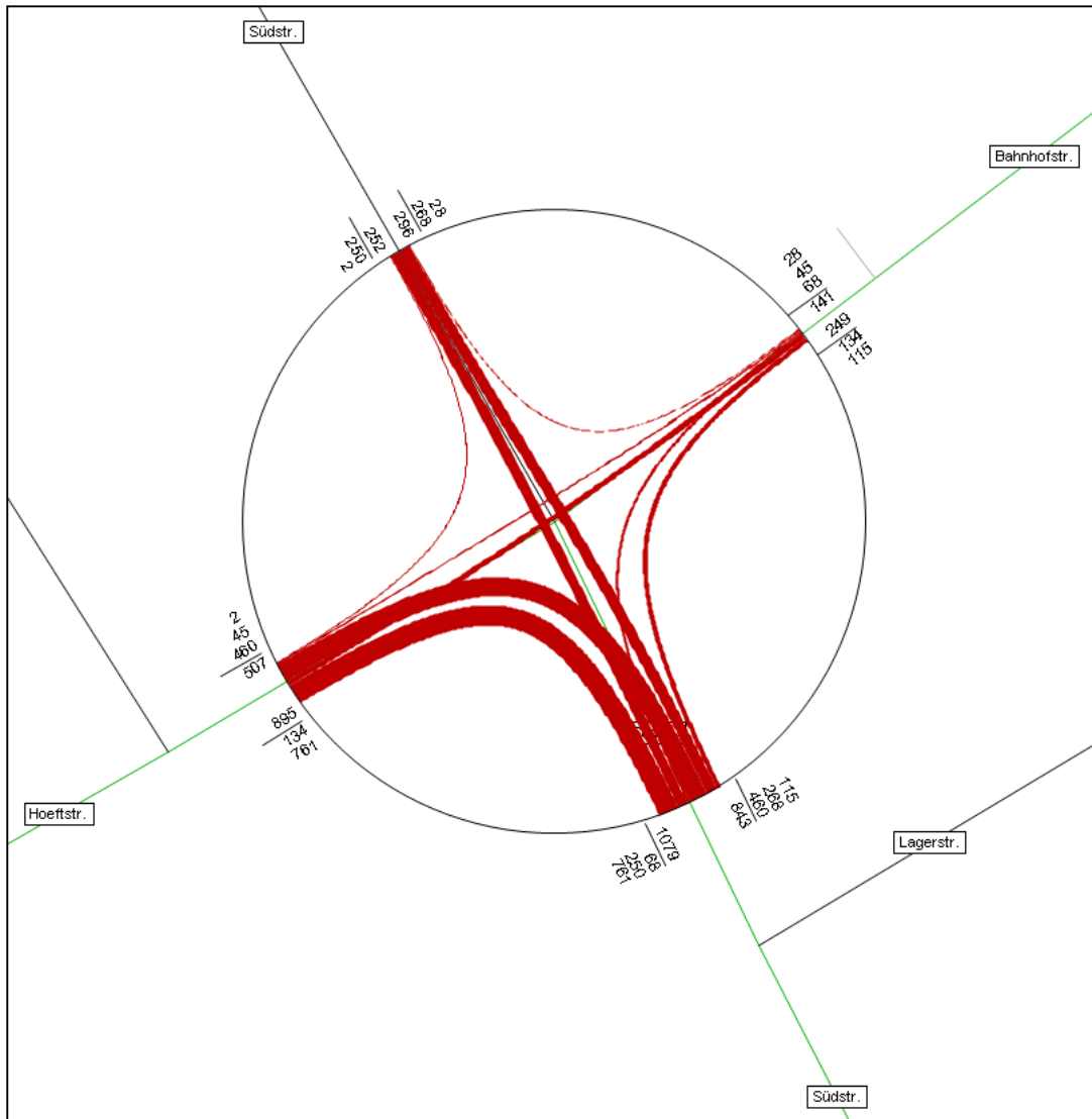
Abbildung 17: Knotenstromdarstellung für LZA 232, Planfall A
