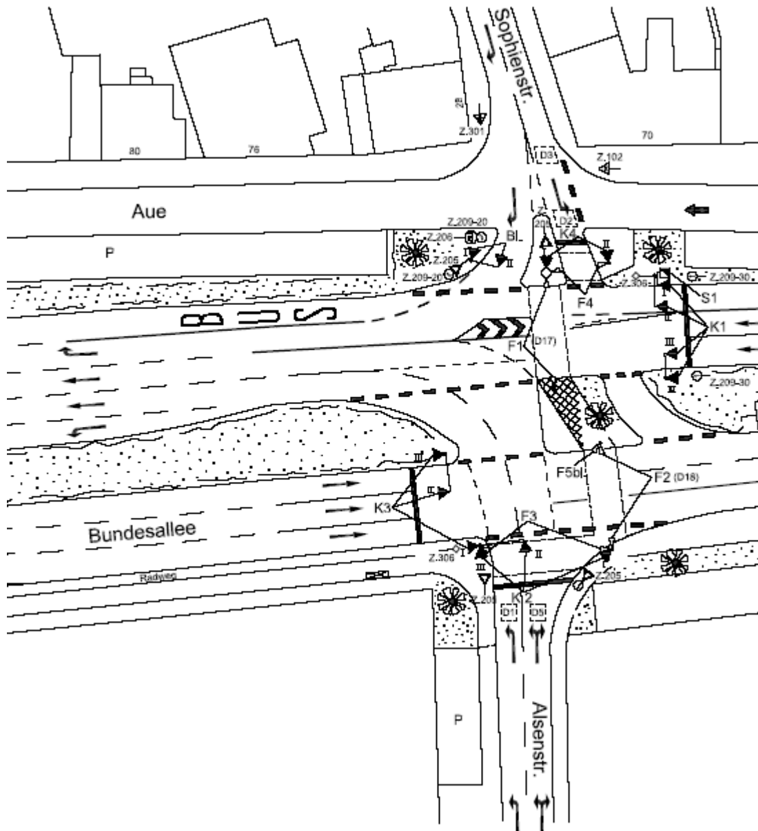
Abbildung 30: Signallageplan LZA 229, Bundesallee (B7)/Alsenstraße/Sophienstraße
