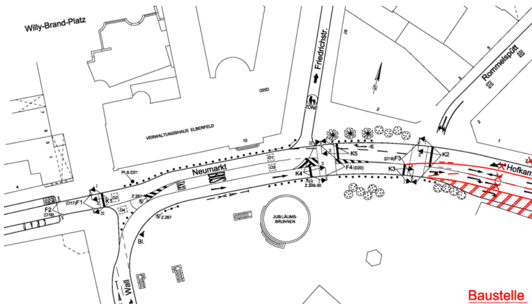
Abbildung 25: Signallageplan LZA 216, Neumarkt/Wall/Rommelspütt (Baustellenzustand Hertie)
